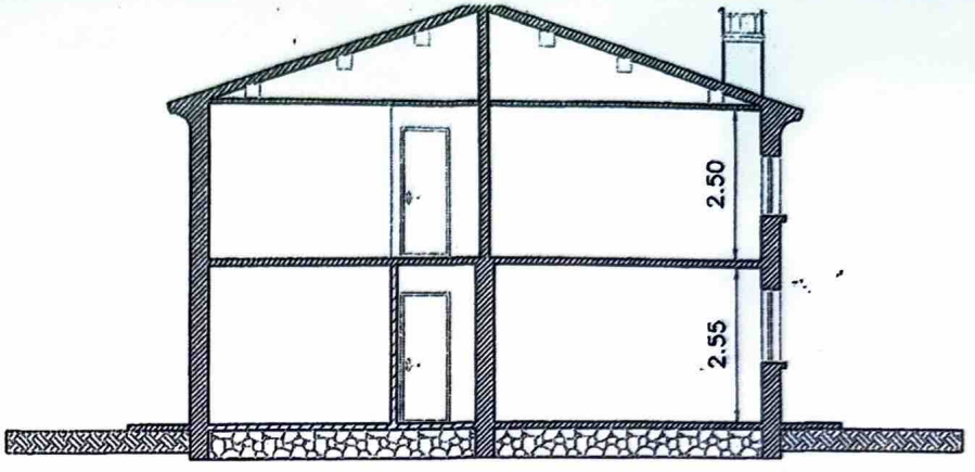
SEZIONE A-A
