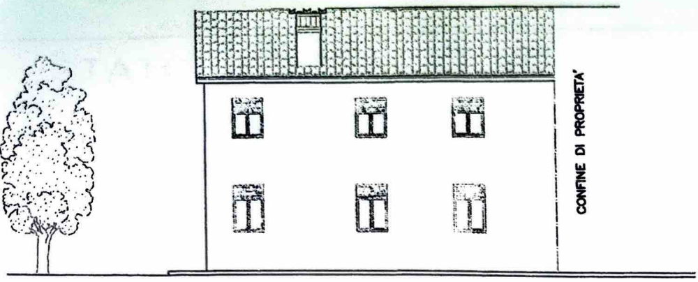
PROSPETTO SUD
